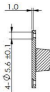
profile A-A
